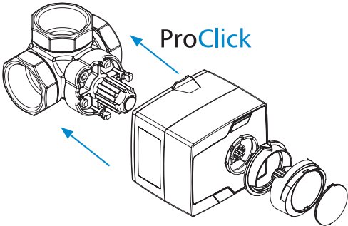
Fig. 5. Système ProClick
