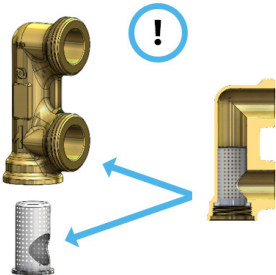
Рис. 15. Правильне розташування сіткового фільтра
