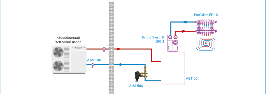
Рис. 13. Приклад схеми монтажу з комплектом сервісної арматури для теплових насосів AHS 560
