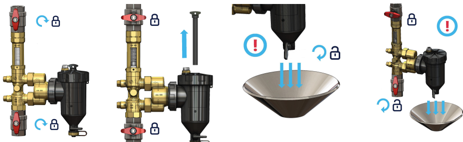
Рис. 16. Схема технічного обслуговування AHS 560
