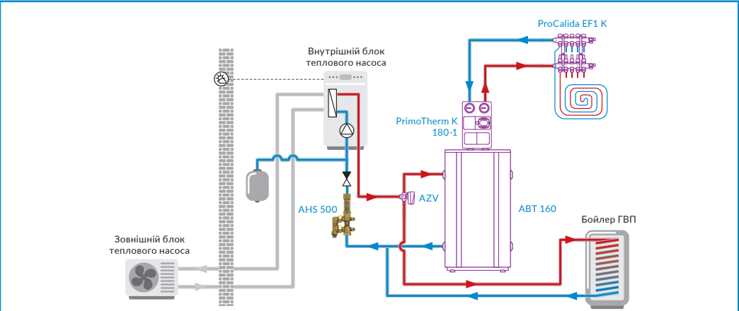
Рис. 12. Приклад схеми монтажу з комплектом сервісної арматури для теплових насосів AHS 500
