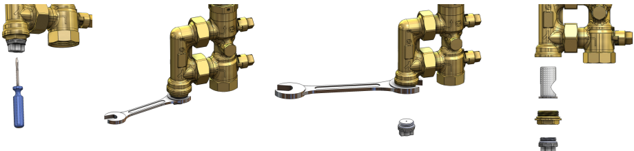
Рис. 14. Схема технічного обслуговування AHS 500
