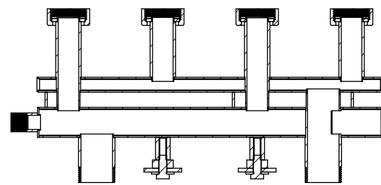
PRZEKRÓJ SKALA 1 : 5
