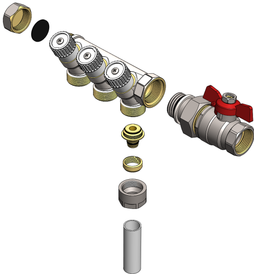
Рис. 5. Примерная схема монтажа балки коллектора для горячей воды с главным соединением с правой стороны
