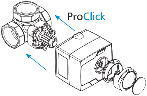
Abb. 5. ProClick-System
