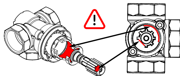
Rys. 2. Położenie zawieradła względem spłaszczenia na adapterze i trzpieniu
