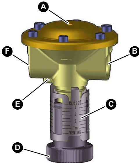
Abbildung 1: Übersicht
