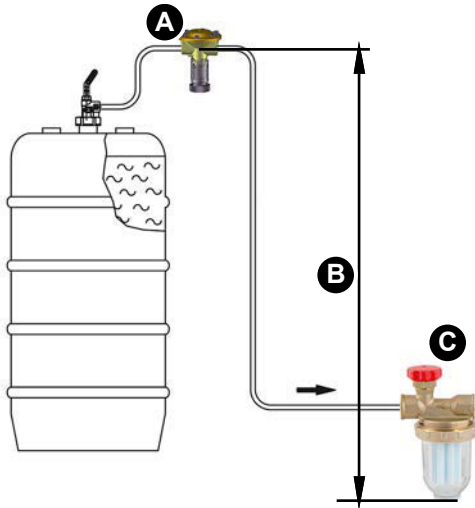
Abbildung 3: Montage vorbereiten
