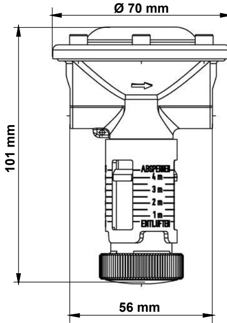
Abbildung 2: Abmessungen
