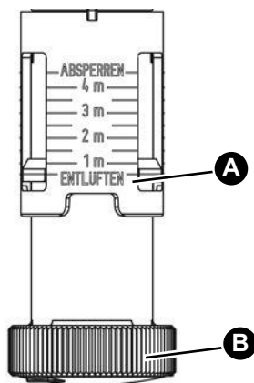
Abbildung 6: Einstellung „Entlüften“
