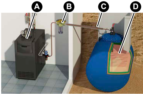
Abbildung 5: Montage bei teilweise selbstsichernder Saugleitung
