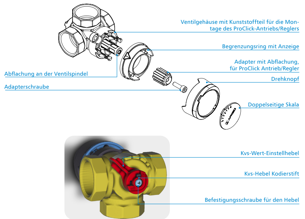
Abb.1. Konstruktion der 3-Wege-Mischventil ARV Vario ProClick
