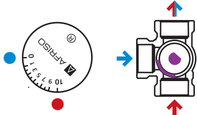
Abb. 3. Position des Zifferblatts mit Skala
