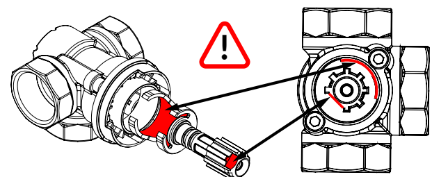
Abb. 2. Position des Verschlusselements in Bezug auf die Abflachung auf dem Adapter und der Ventilspindel
