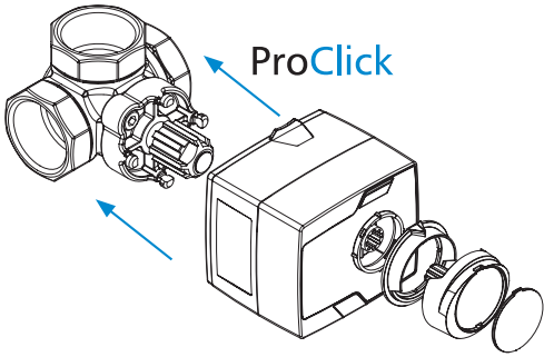
Abb. 5. ProClick-System
