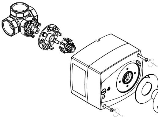
Рис. 2. Монтаж приводу ARM/контролера ACT
