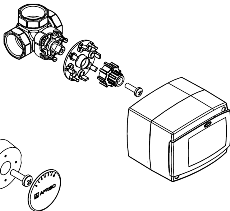
Рис. 3. Монтаж контролера ACT
