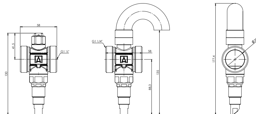
Rys. 2. Wymiary zaworu AAV 300
