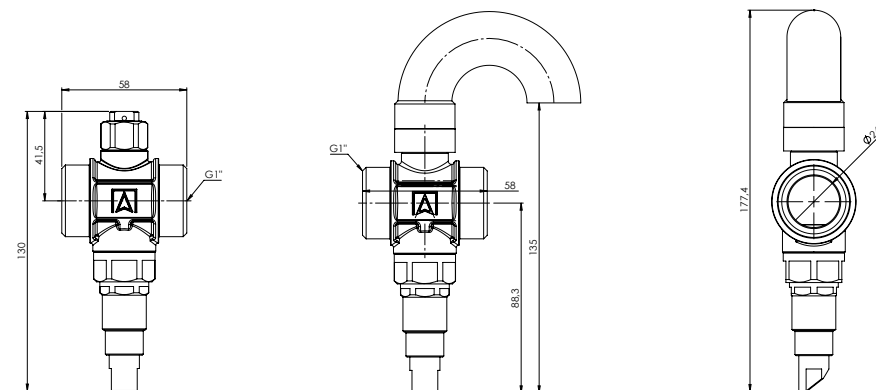
Rys. 1. Wymiary zaworu AAV 100
