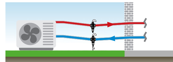
Rys. 7. Dopuszczalna pozycja montażowa zaworów z osłonami
