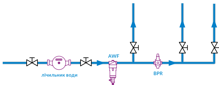
Рис. 2. Прикладова схема застосування редуктора BPR у системі
