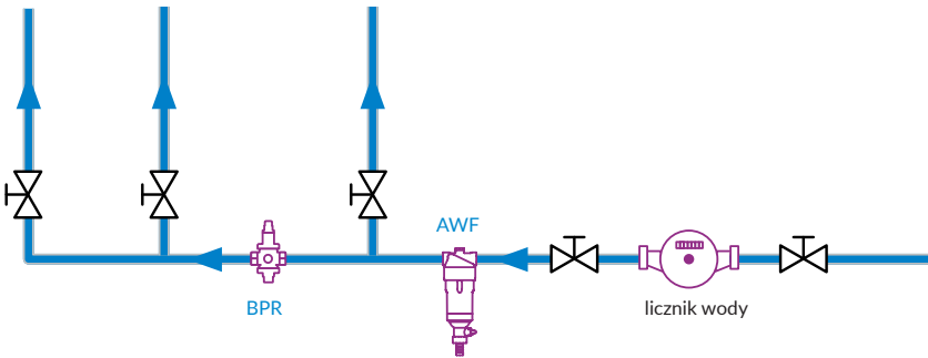
Rys. 7. Przykładowy schemat montażu filtra AWF
