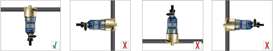
Rys. 5. Dopuszczalna pozycja montażowa filtrów AWF
