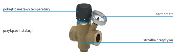
Rys. 1. Budowa zaworu ATB 100 i ATB 110 (bez funkcji przegrzewu)
