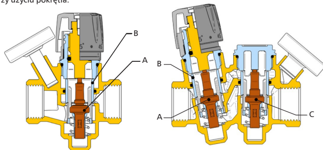
Rys. 3. Konstrukcja wewnętrzna zaworów ATB. Po lewej stronie ATB 100 i 110, po prawej stronie ATB 200 i 210
