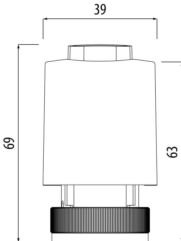
Rysunek wymiarowy
