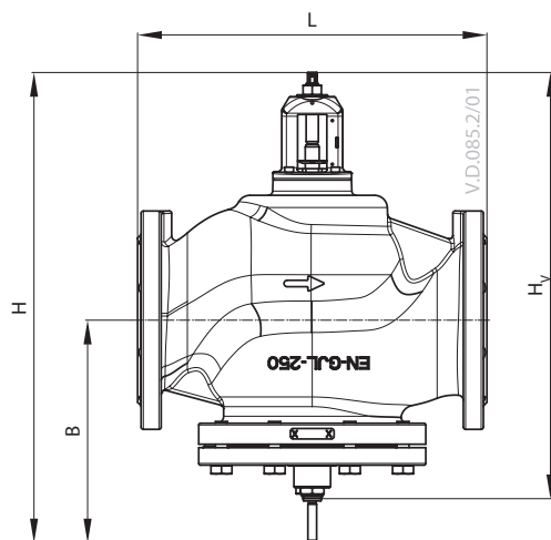
VFQ 22(1) DN 65-250
