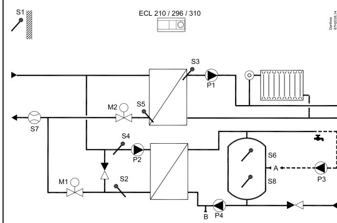
Typowa aplikacja A247.2, przykład a:
