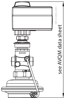
AMV 10, AMV 11 + AVQM PN 25
