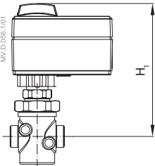
AMV 10, AMV 11 + VM 2 (DN 15-32)
