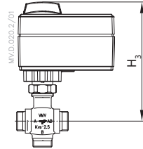
AMV 10, AMV 11 + VMV (DN 15-40)
