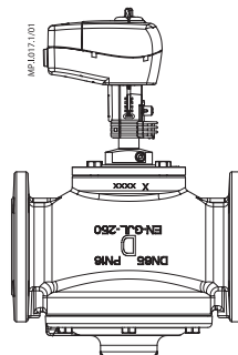
AMV(E) 435 + AHQM DN 50
