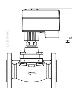
AME 13 + VB 2 (DN 15-25)
