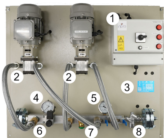
Rys. 2. Budowa agregatu RL wiszącego z dwiema pompami.
