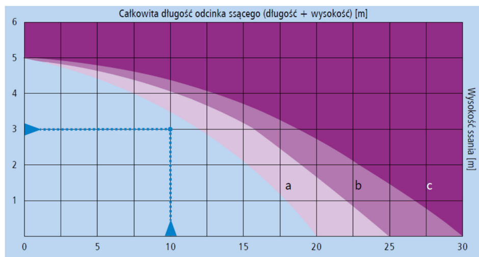
Rys. 3. Wykres doboru agregatu pompowego.
