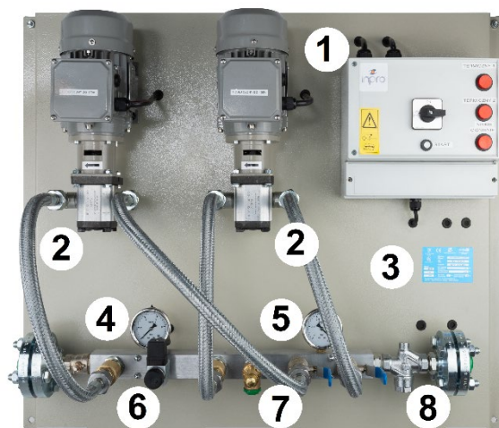
Rys. 2. Budowa agregatu FP 2-pompowego wyposażonego w presostat.
